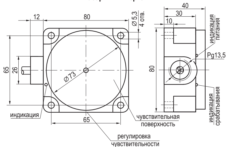
Габаритный чертеж
